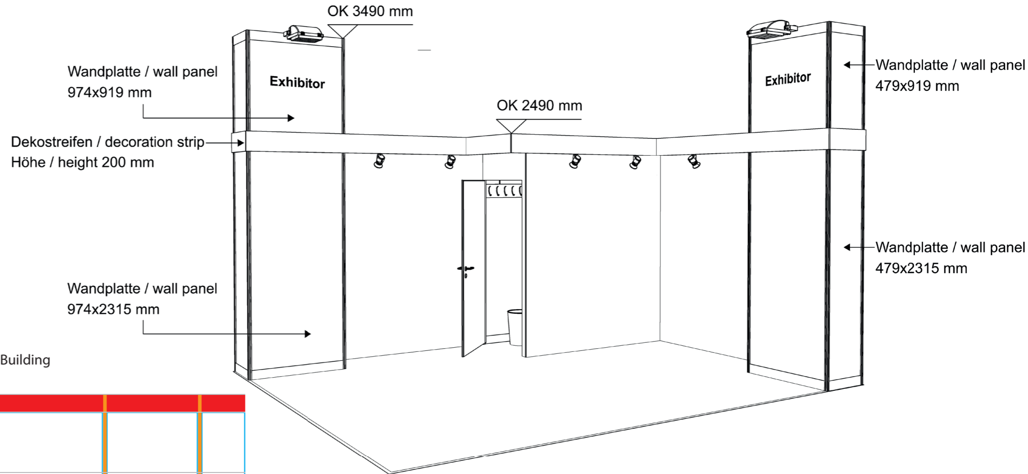
Beispiel/Sample Eckstand/Cornerstand 4x5m
